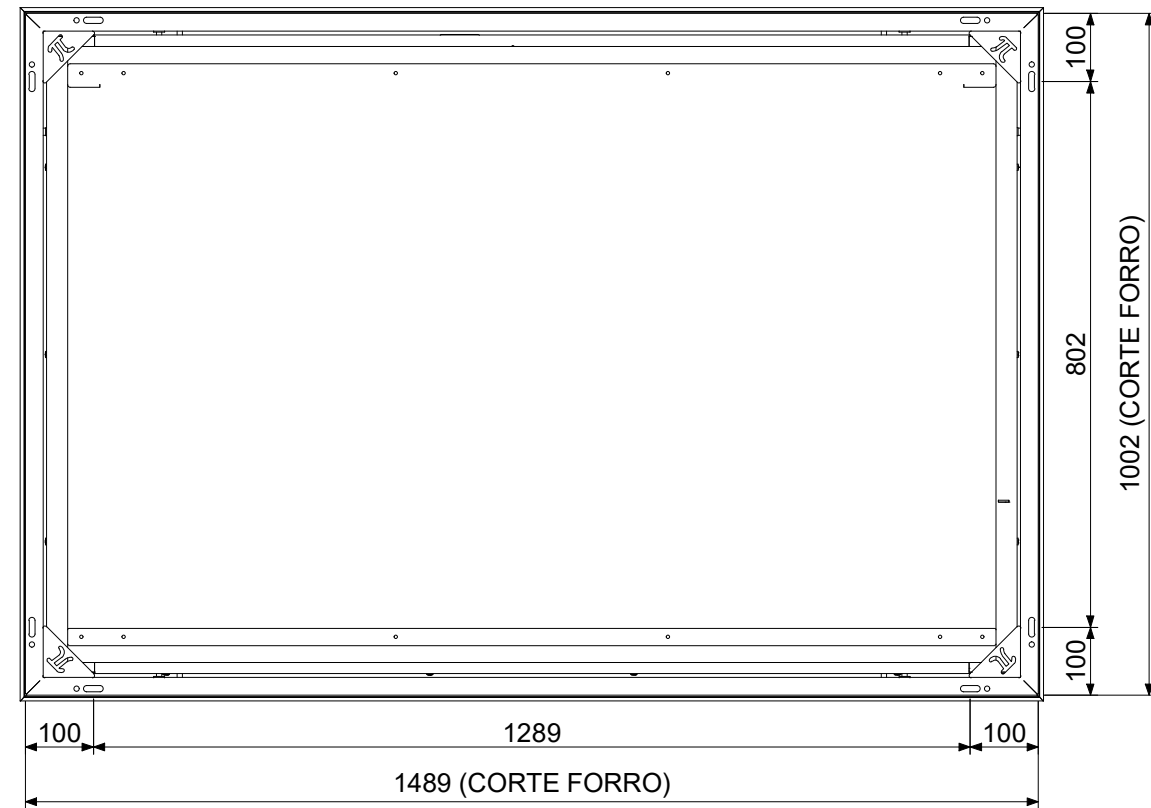
FRENTE VISTA SUPERIOR
