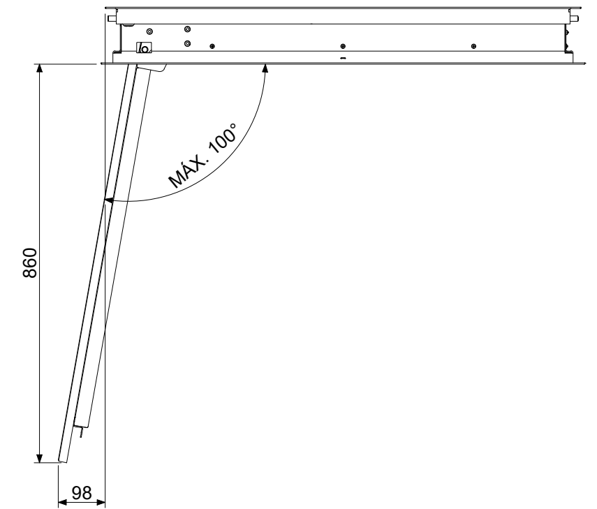
VISTA LATERAL ABERTO
